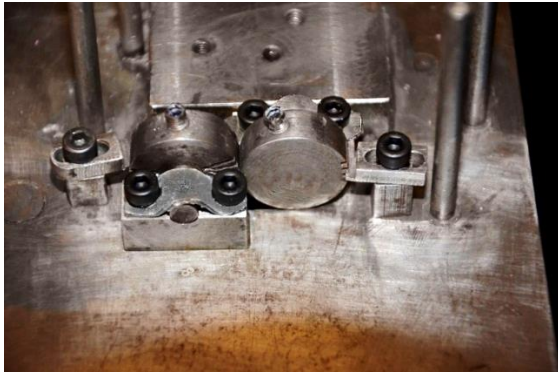
شکل ۳: ایمپلنت هولدر دستگاه مورد استفاده
